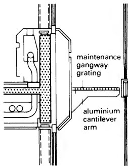
5 Maintenance gangway
